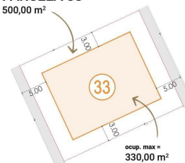
PARCELA 33 500,00 m 2
